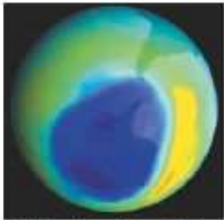
An toull er gwiskad ozon d'ar brasañ m'eo bet e 2000, a-us da Antarktika.
